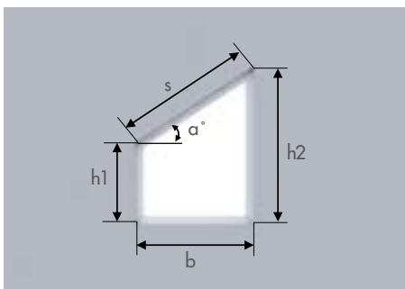
Fenêtre oblique (côté supérieur) - modèle 5
