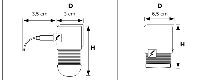
Inbouwdiepte incl. steun en bediening ( D ) Pakke hoogte ( H )
