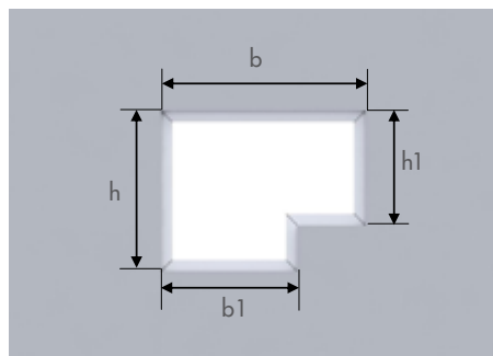
Raam/deurcombinatie - model 2
