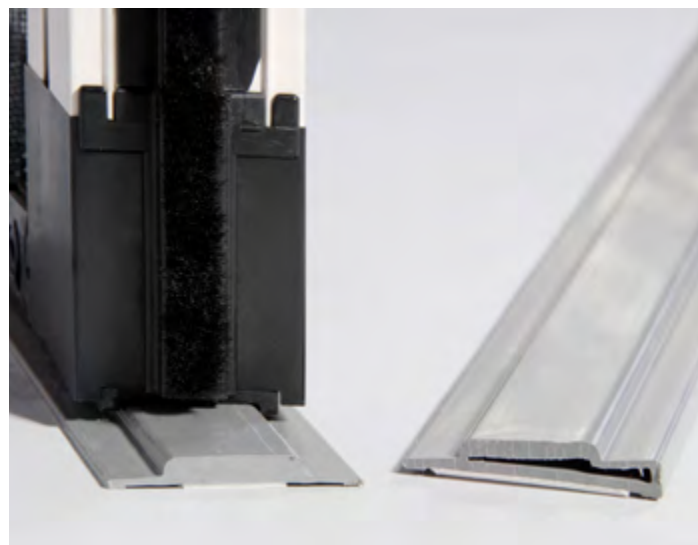
Rechte en schuine ondergeleider
