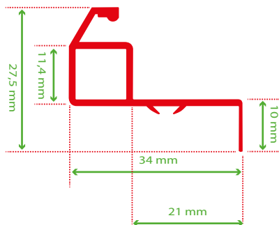
Standaard profiel 34 mm
