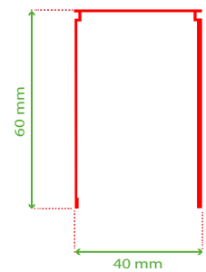
Bovenprofiel
