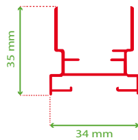
Vast profiel smalle deur
