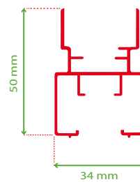
Vast profiel brede deur
