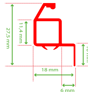
Smal profiel 18 mm
