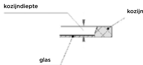
Doorsnede voor de kozijndiepte
