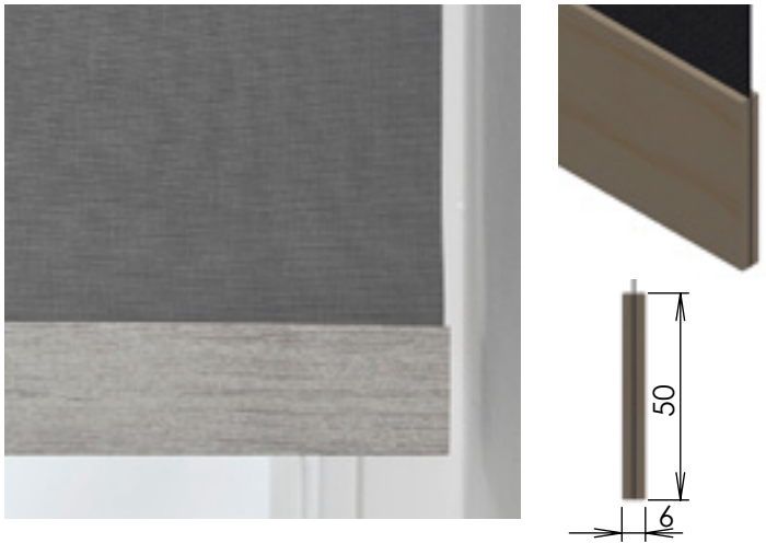
Houten onderlat HL4
