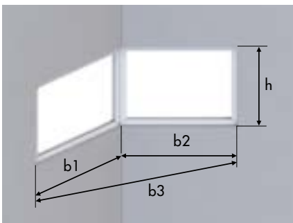
Fenêtre de coin - modèle 6
