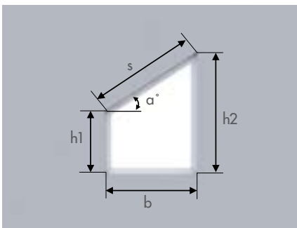
Fenêtre oblique (partie supérieure) - modèle 5
