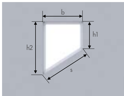
Fenêtre oblique (partie inférieure) - modèle 11
