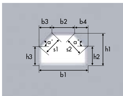
Modèle en arc, rail plié deux fois - modèle 9
